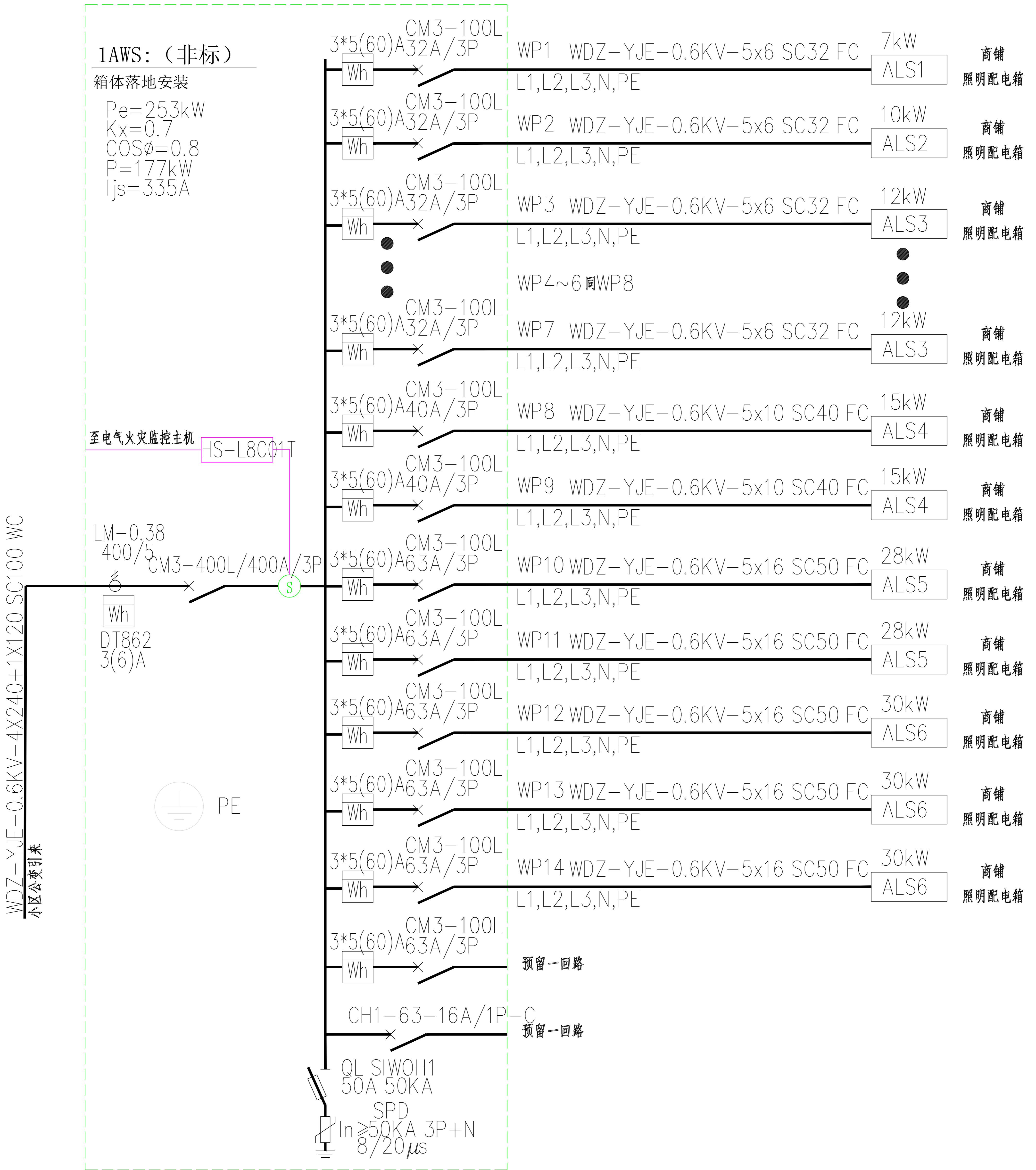
3#、4#楼商铺电表箱系统图1
